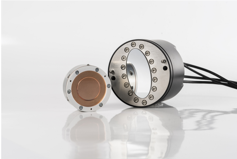
Abbildung 3: Adaptive Fokussierspiegel mit kürzesten Reaktionszeiten. Links: Ausführung mit integrierter Planfeldkorrektur für Applikationen in Laserstrukturierungsanlagen. Rechts: Ausführung für Laserschneiden/Laserschweißen. © Fraunhofer IOF
