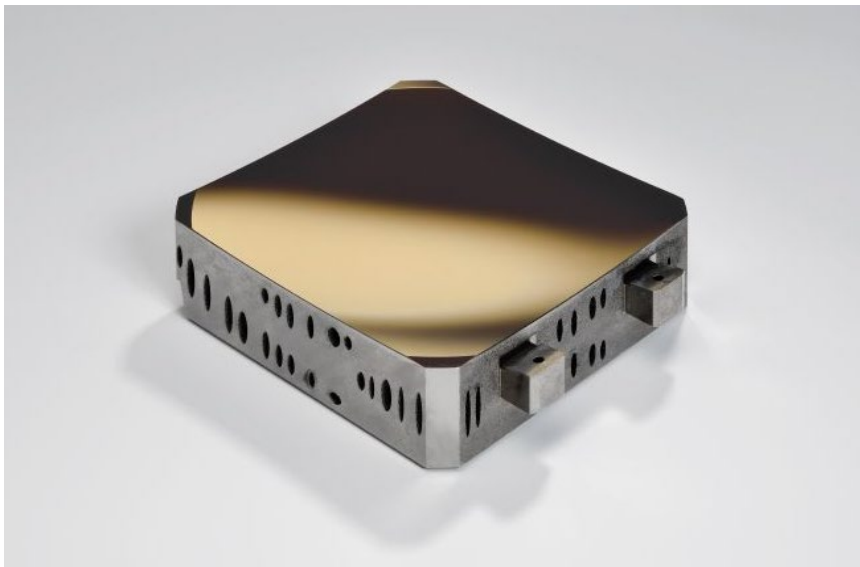
Abbildung 1: Additiv gefertigte Leichtgewichtspiegel aus AlSi-Legierung nach Beschichtung mit geschütztem Silber. © Fraunhofer IOF
